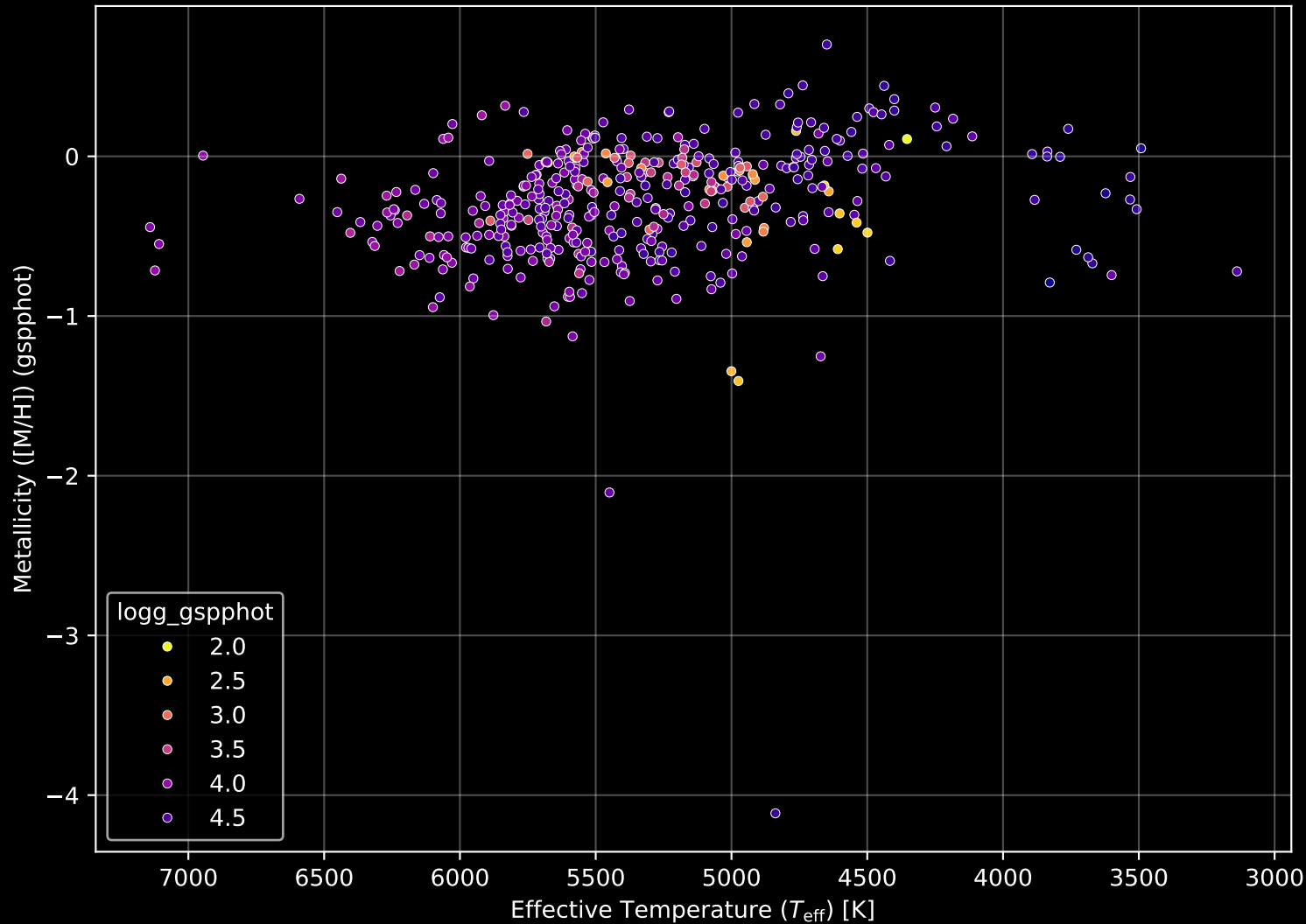
GALAH DR4 Field: [6575] Stellar Population Parameters (n= 427)
