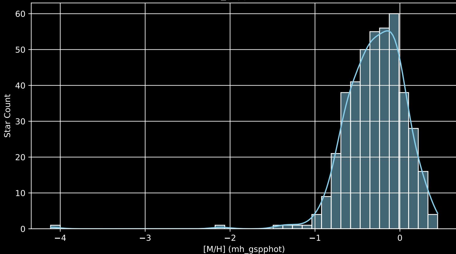
GALAH DR4 Field: [6575] [M/H] (mh_gspphot) (n= 426)
