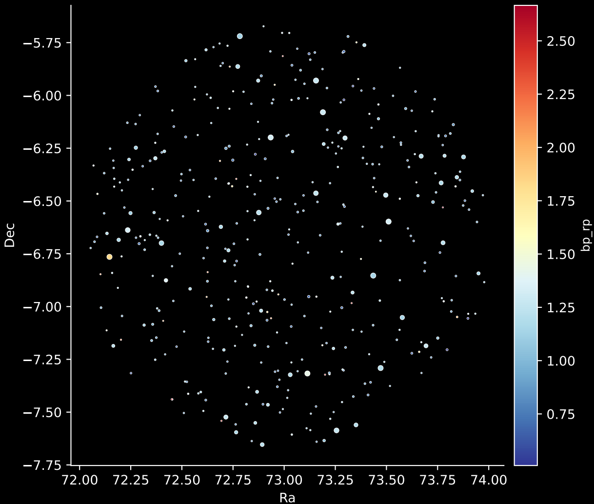
GALAH DR4 Field: [6575] Stars: 427
